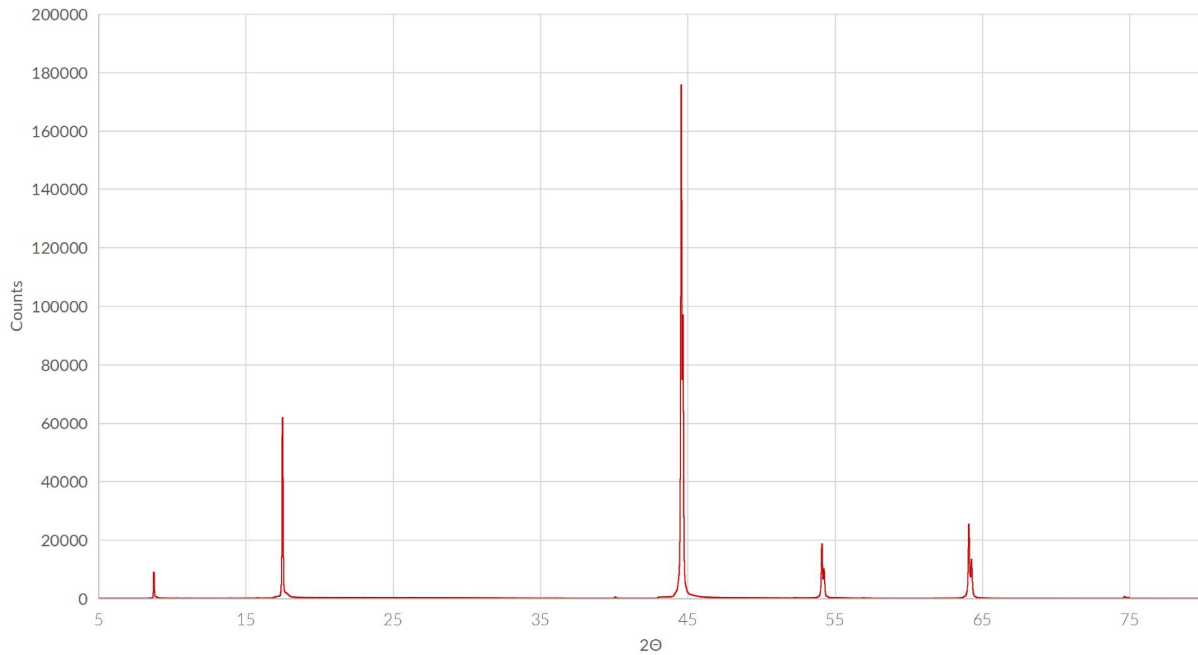
Bi 2 Te 3 , XRD Spectrum (Batch 2017/001)
