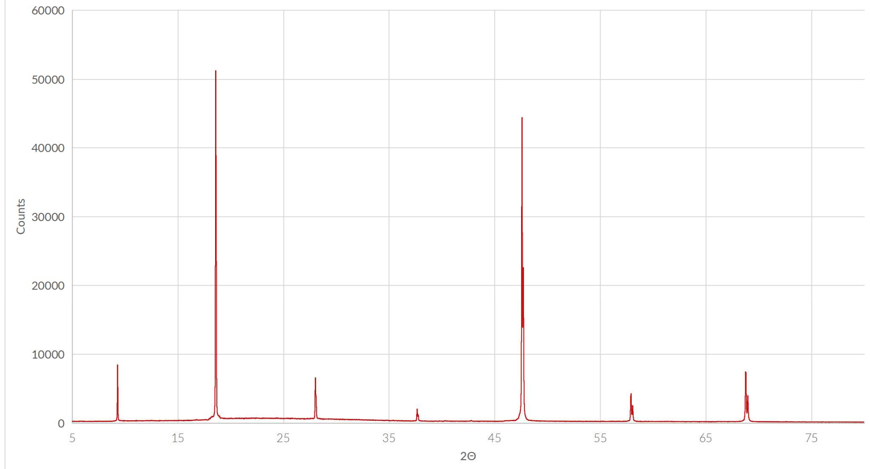
Bi 2 Se 3 , XRD Spectrum (Batch 2017/001)
